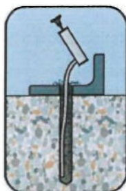
Bohrloch reinigen
